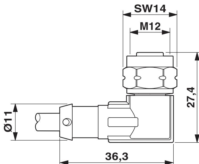
Disegno quotato
