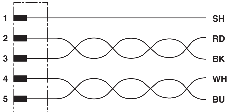
Schema di collegamento
