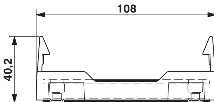
Disegno quotato
