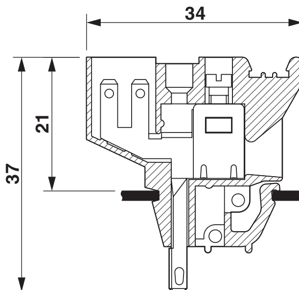
Disegno quotato
