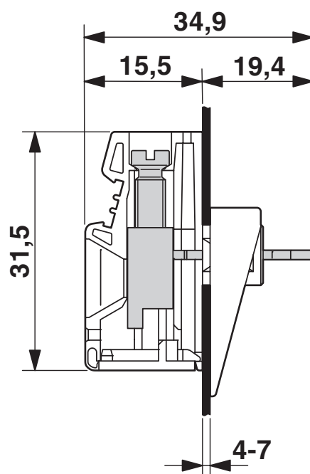
Disegno quotato
