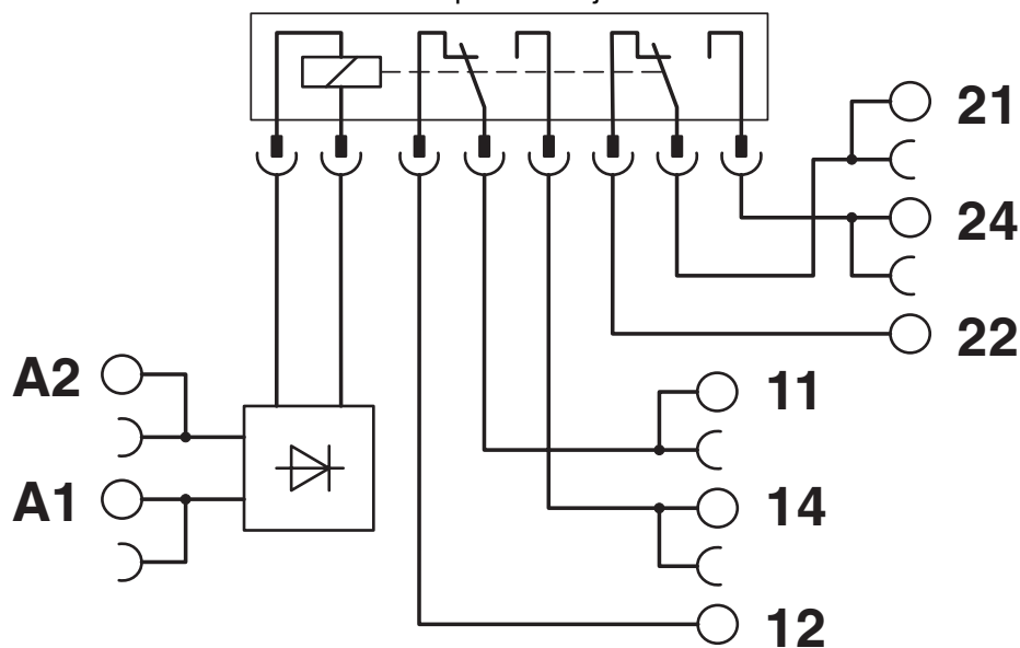
Kapcsolási rajz
