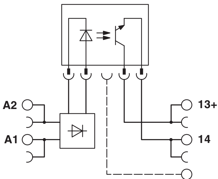
Kapcsolási rajz
