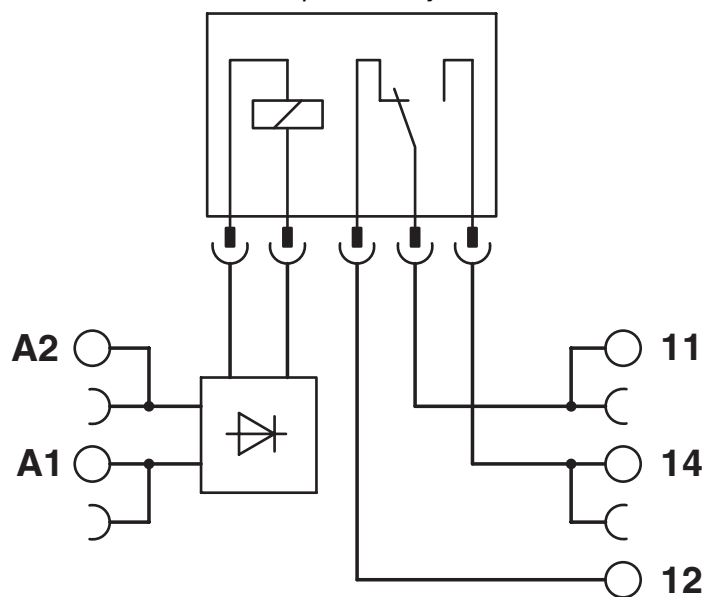
Kapcsolási rajz
