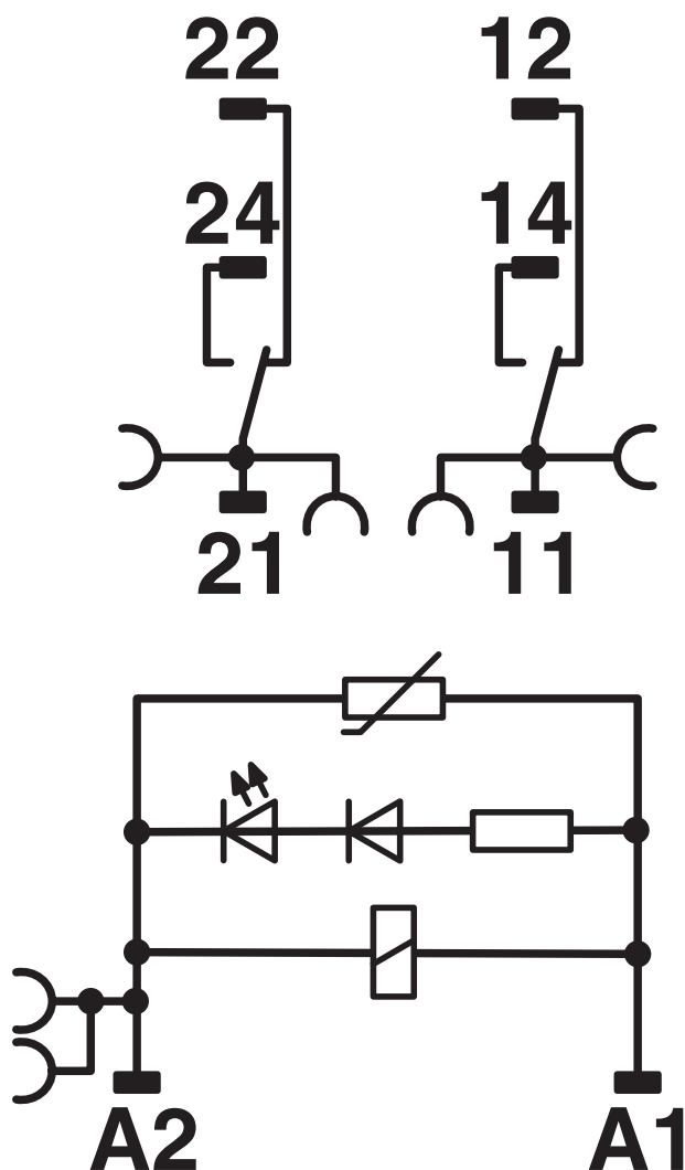
Kapcsolási rajz
