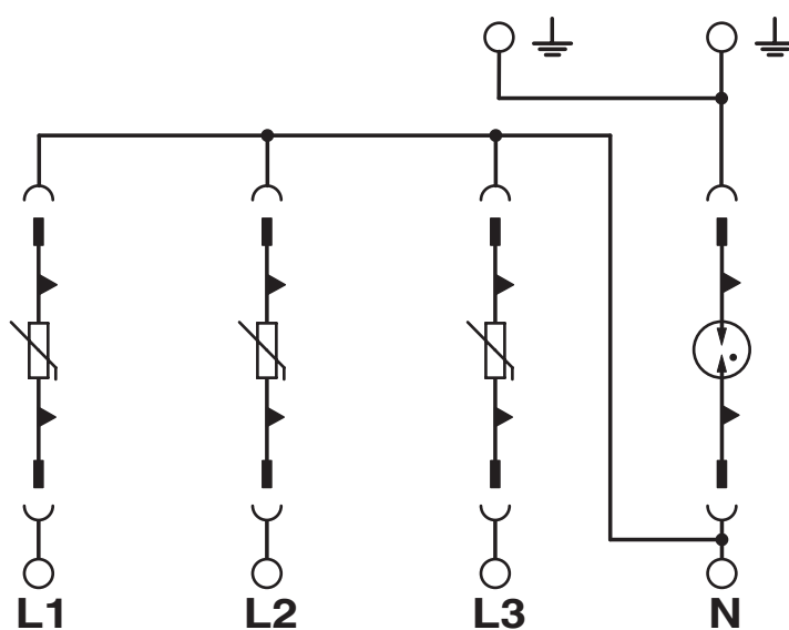
Kapcsolási rajz
