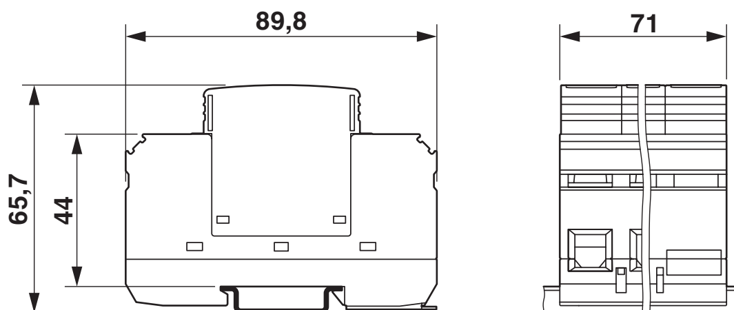
Méretrajz
