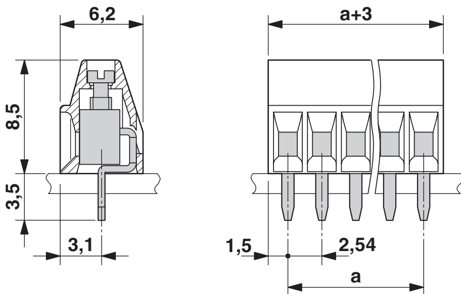
Méretrajz
