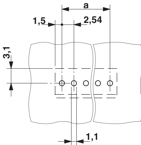
Furatterv/forrasztópád-geometria
