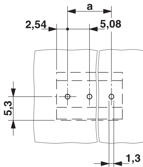
Furatterv/forrasztópad-geometria
