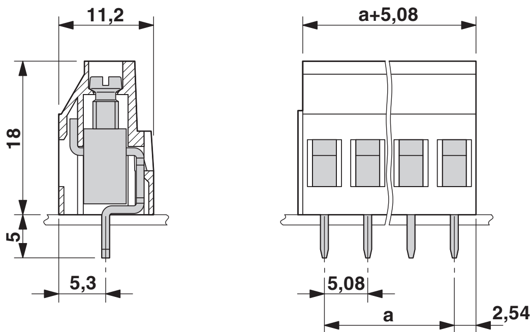
Méretrajz
