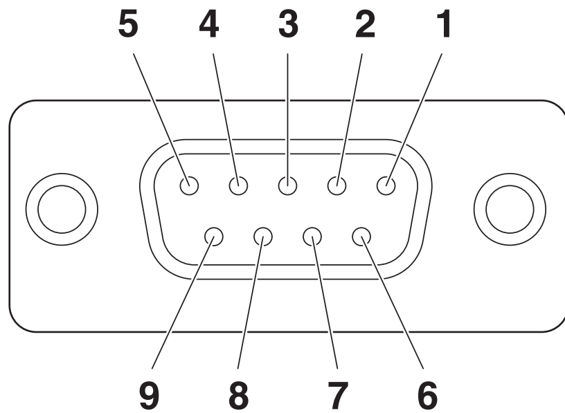
Sematikus rajz
