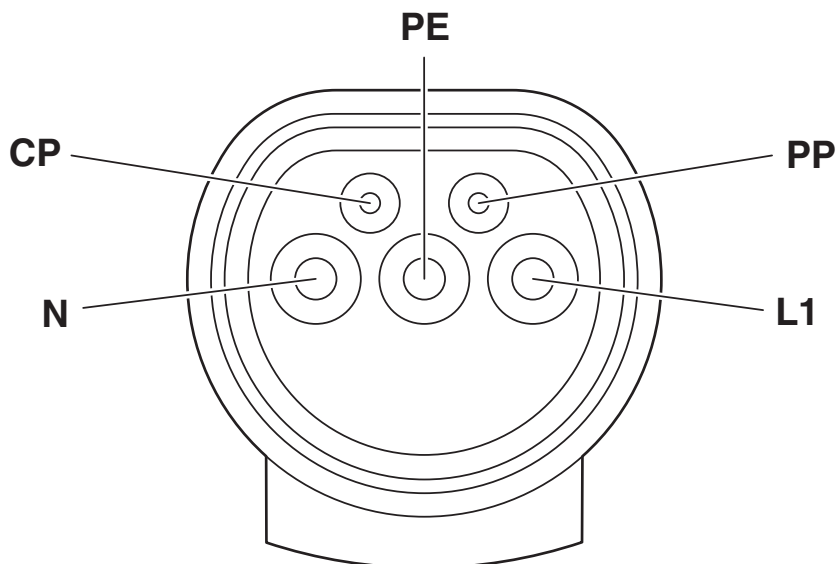
Sematikus rajz
