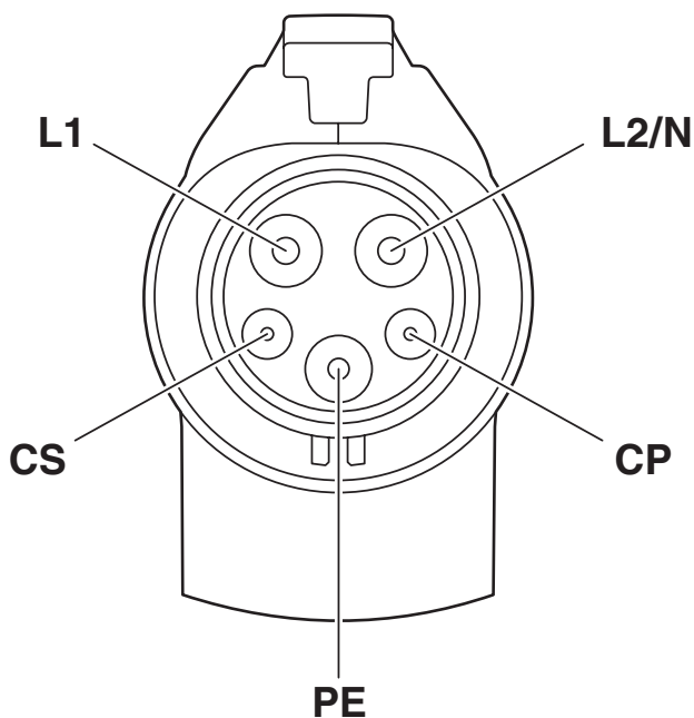
Csatlakozási rajz
