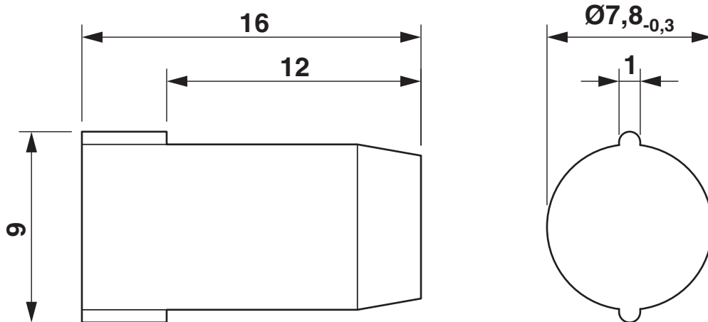
Méretrajz
