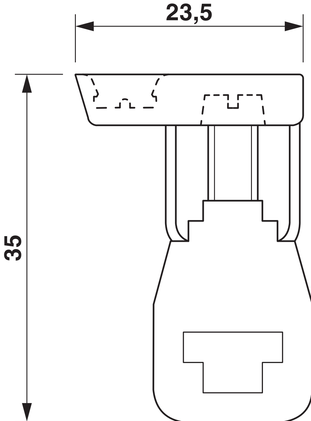
Méretrajz
