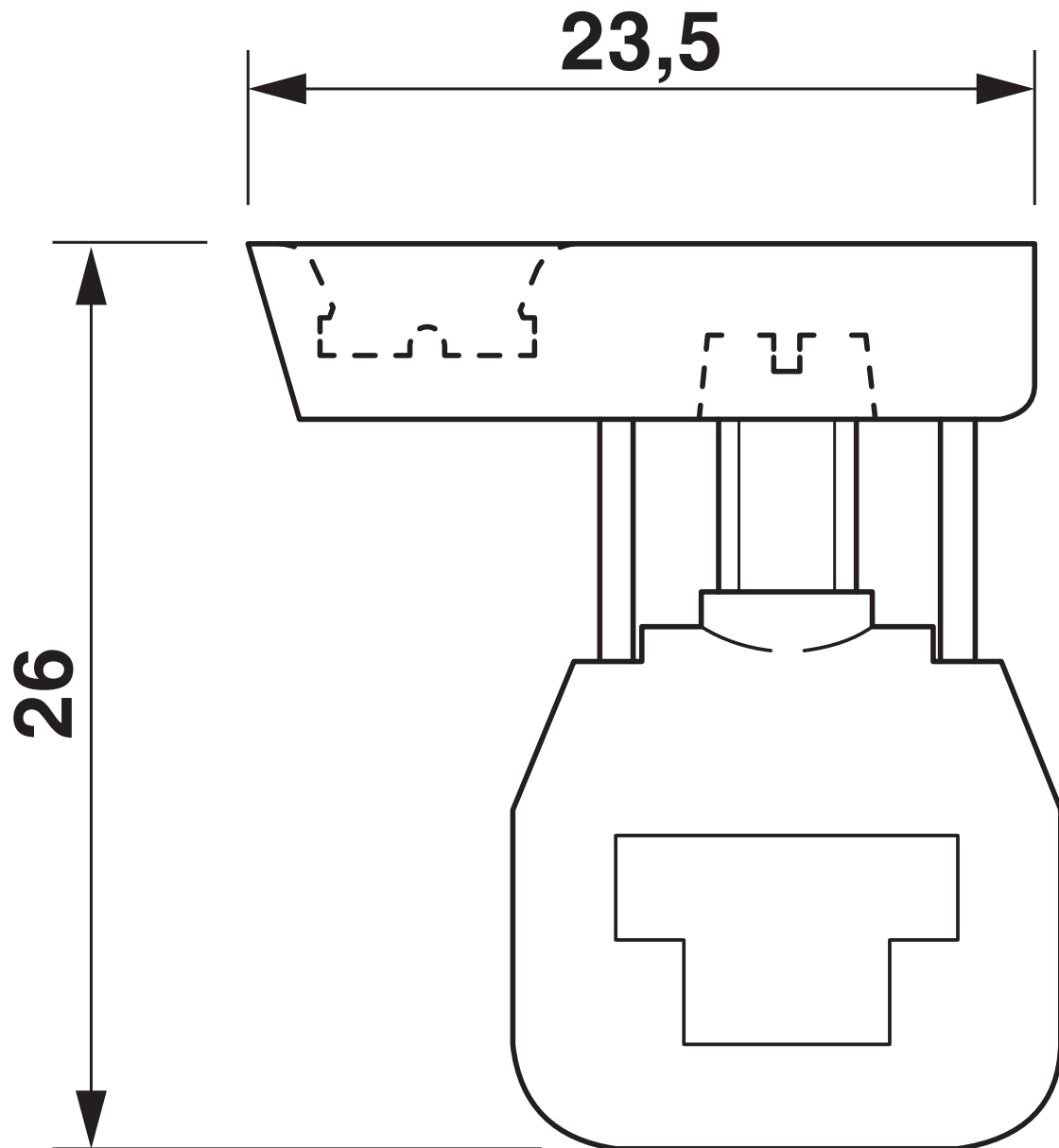
Méretrajz
