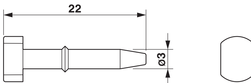
Esquema de dimensiones
