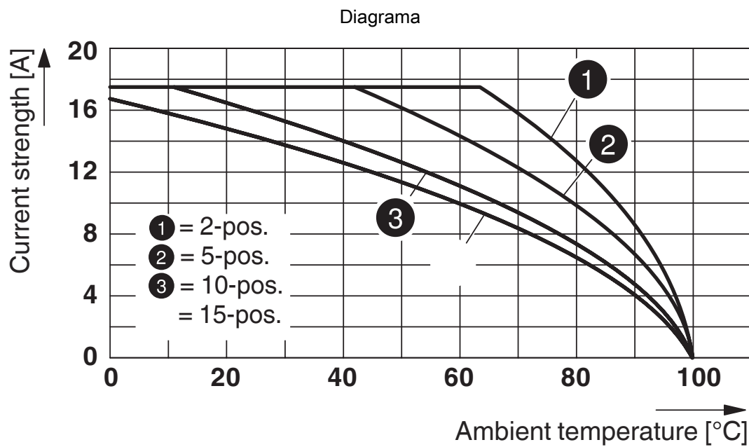
Diagrama eléctrico
