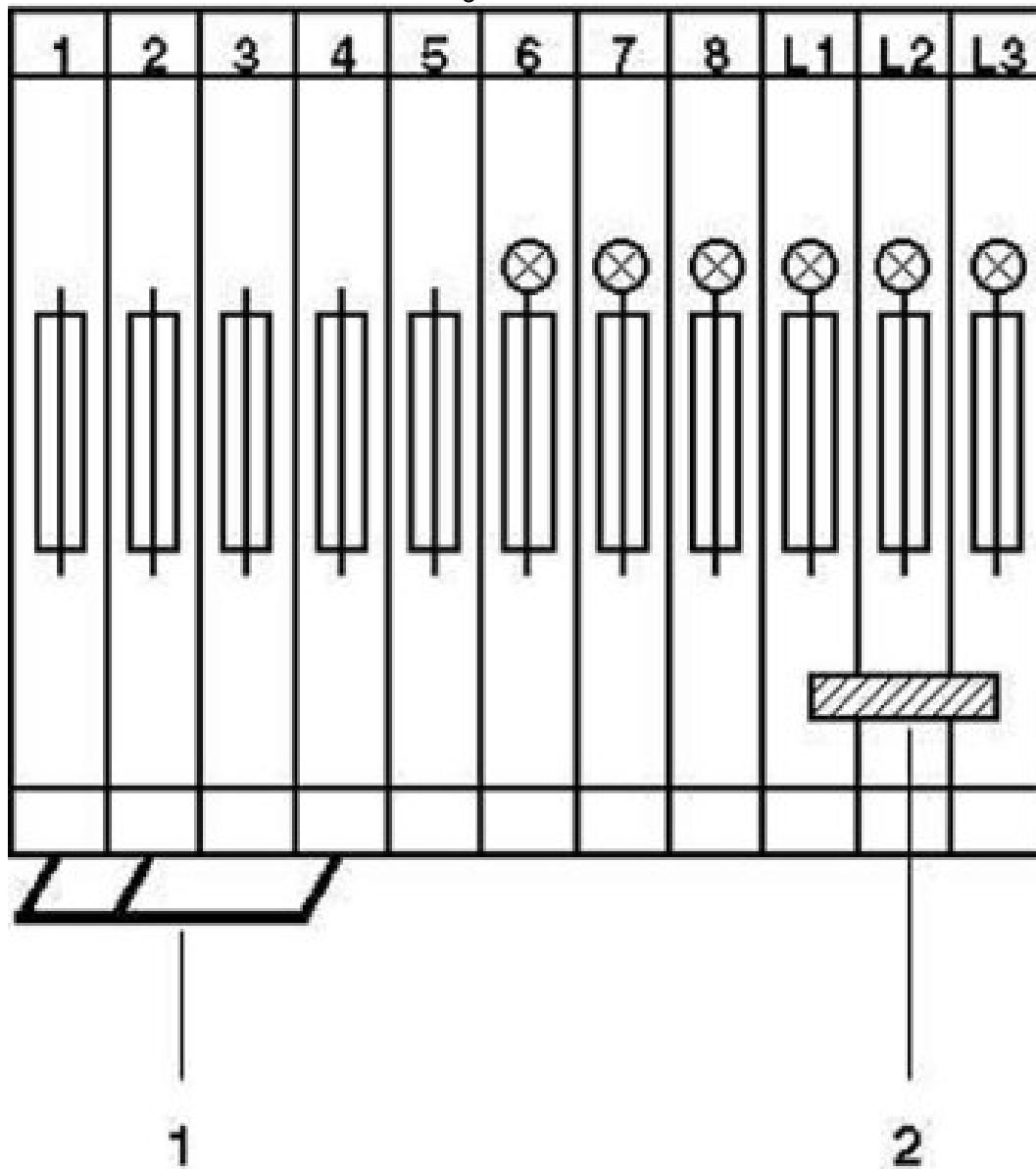
Diagrama eléctrico
