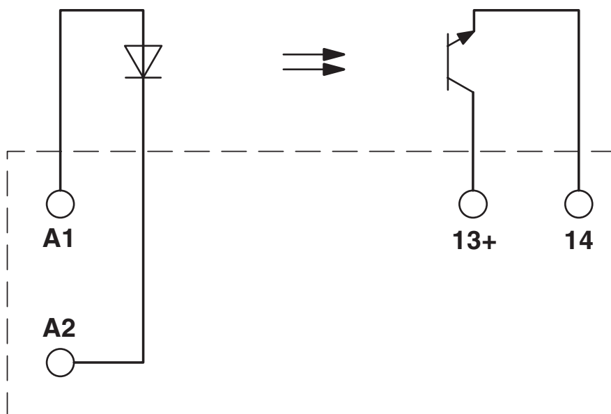
Diagrama eléctrico
