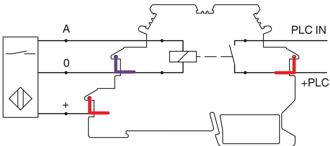
Ocupación de conexiones DEK-REL-...SEN
