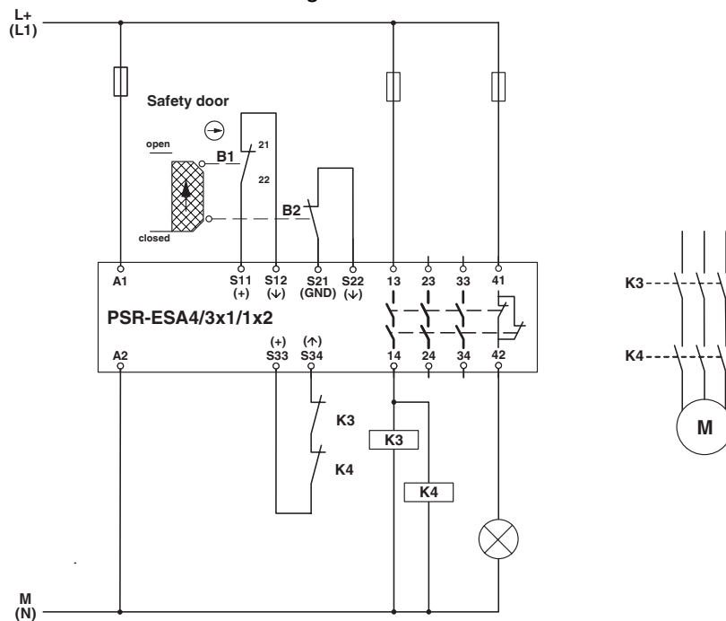
Diagrama eléctrico
