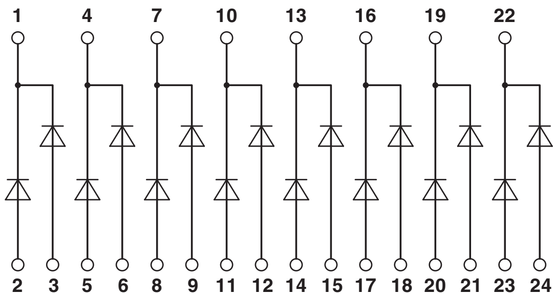
Diagrama eléctrico
