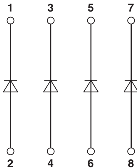
Diagrama eléctrico
