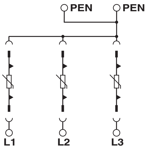
Diagrama eléctrico
