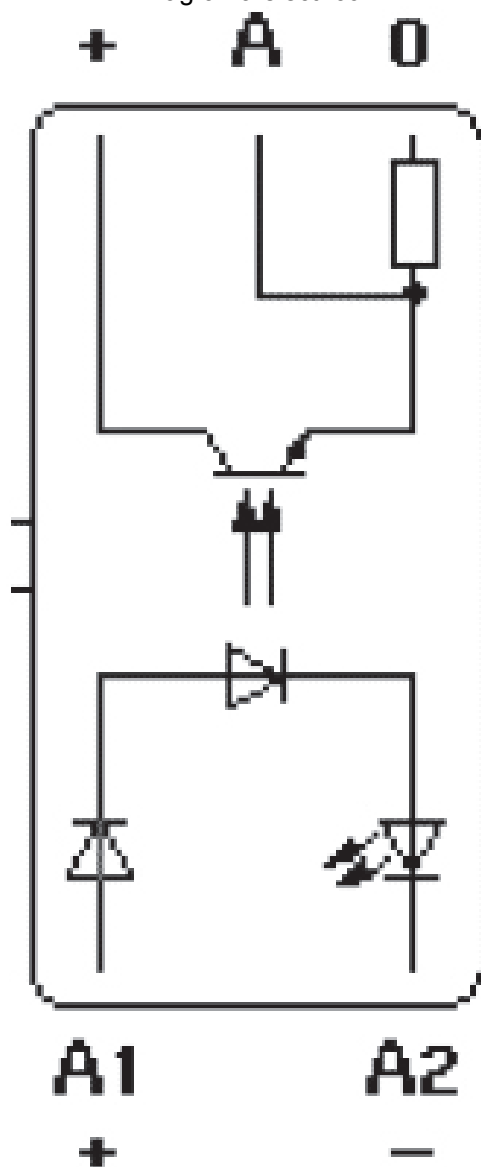
Diagrama eléctrico
