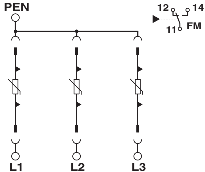
Diagrama eléctrico
