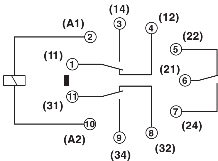
Diagrama eléctrico
