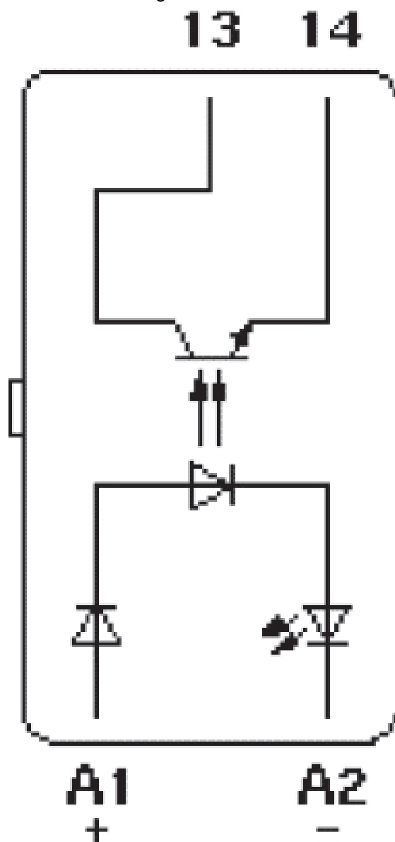
Diagrama eléctrico
