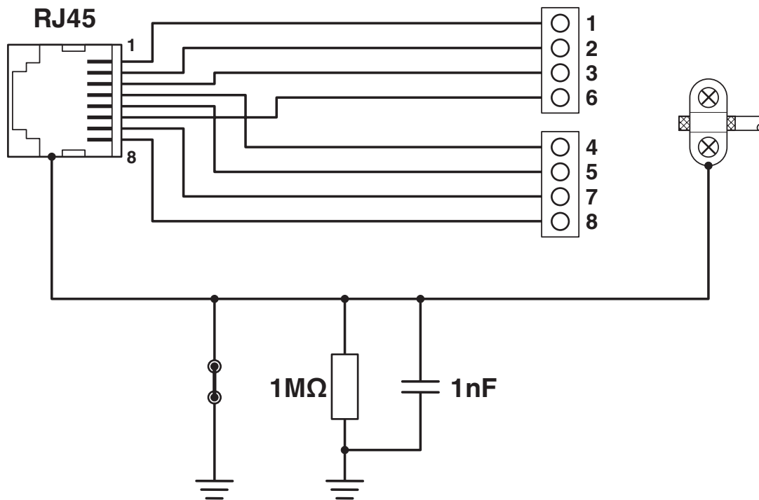
Diagrama eléctrico
