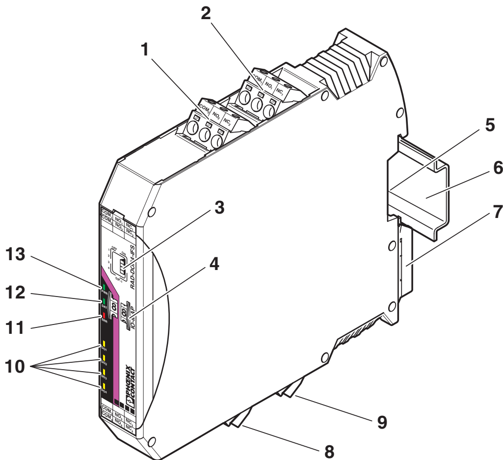
Plano esquemático
