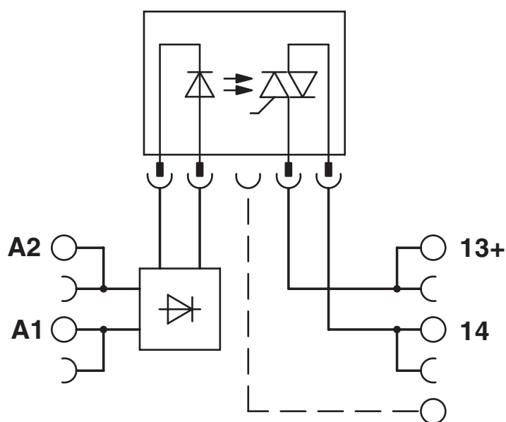
Diagrama eléctrico
