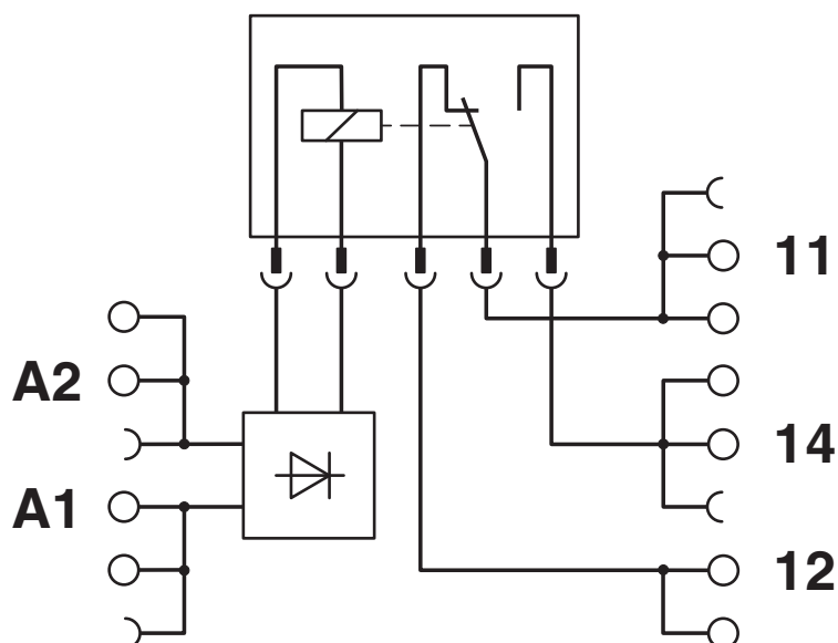
Diagrama eléctrico
