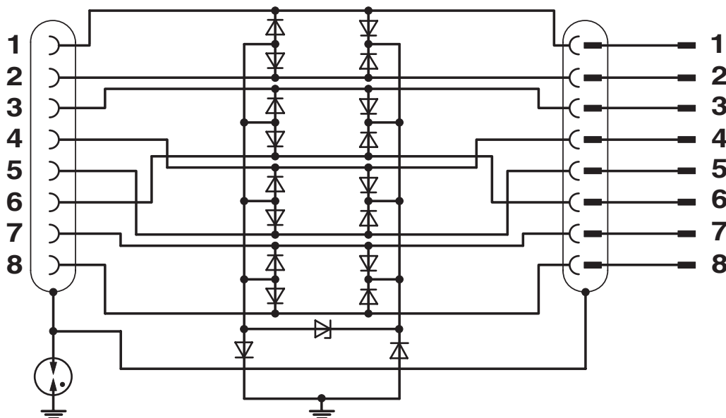
Diagrama eléctrico
