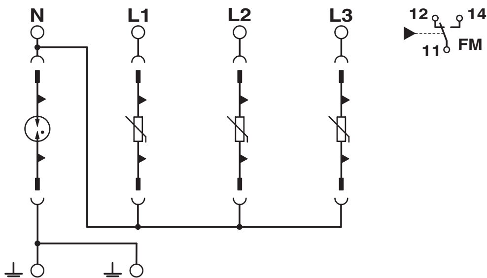
Diagrama eléctrico
