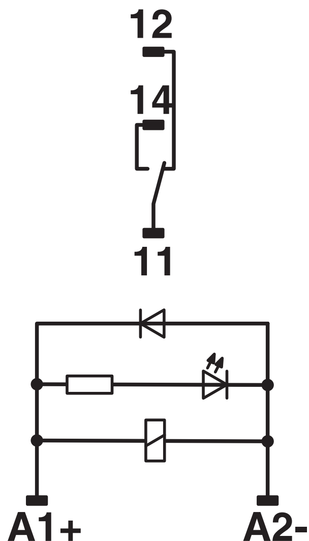
Diagrama eléctrico
