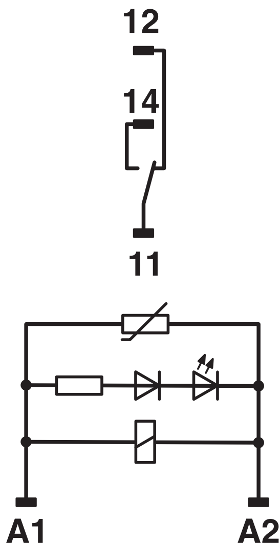
Diagrama eléctrico
