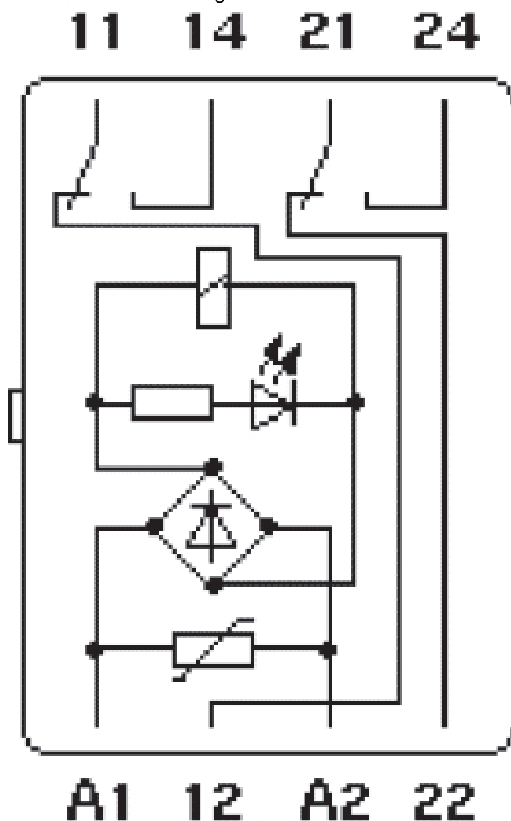
Diagrama eléctrico
