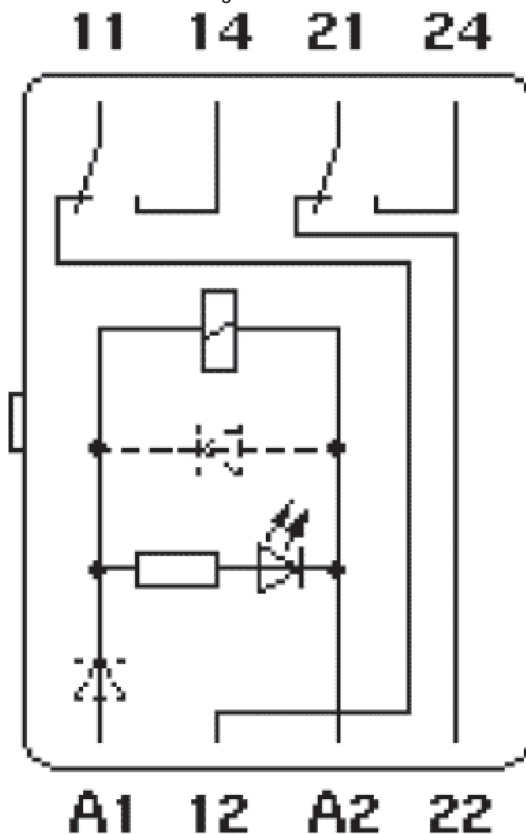
Diagrama eléctrico
