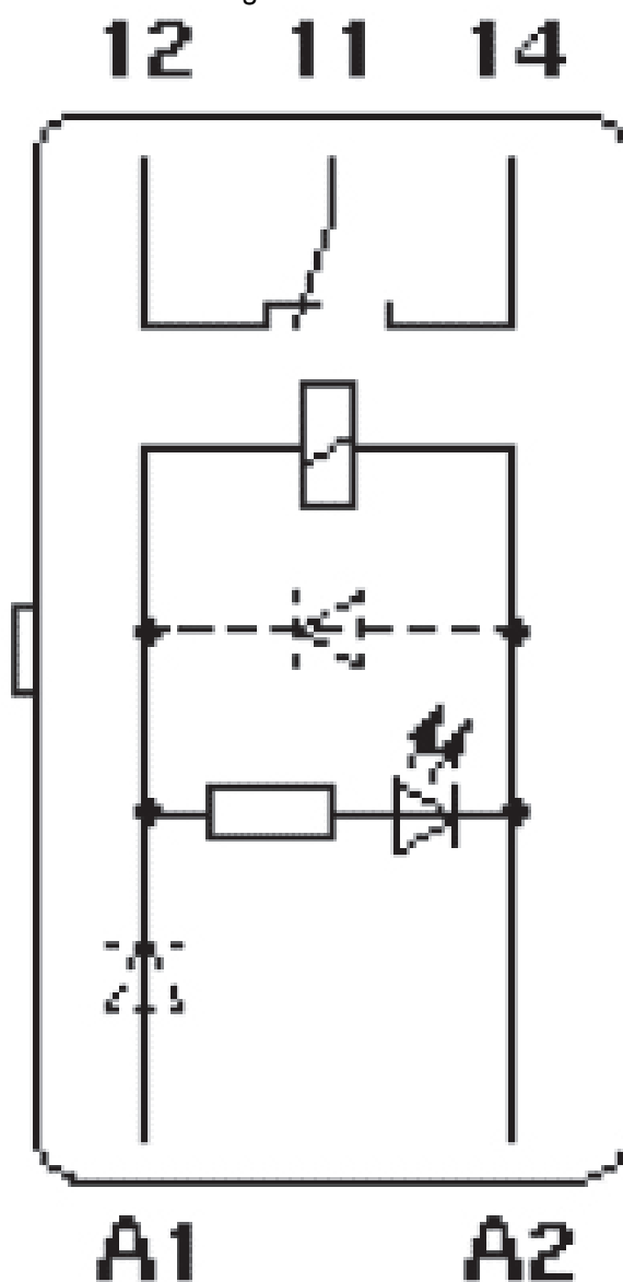
Diagrama eléctrico
