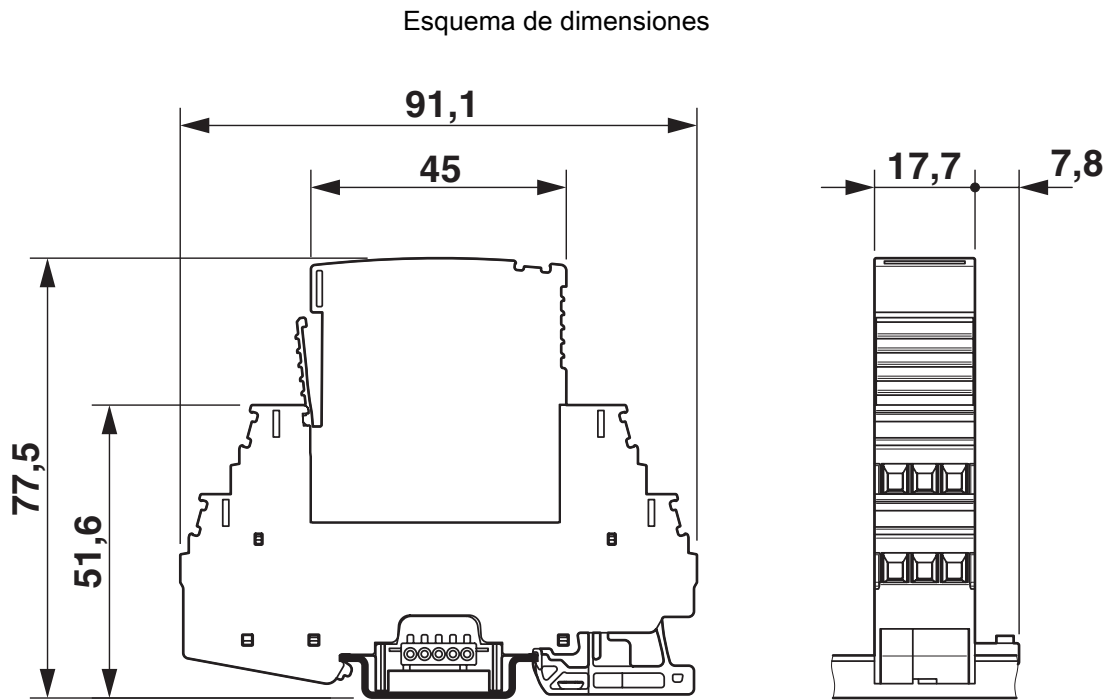
Plano esquemático
