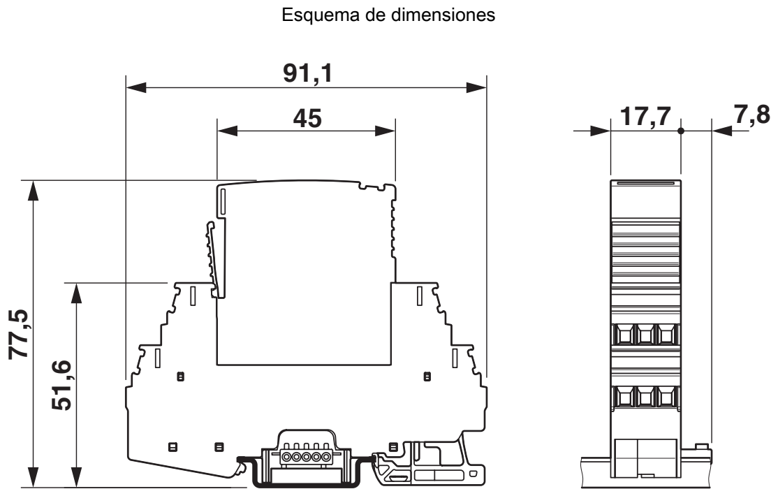
Plano esquemático
