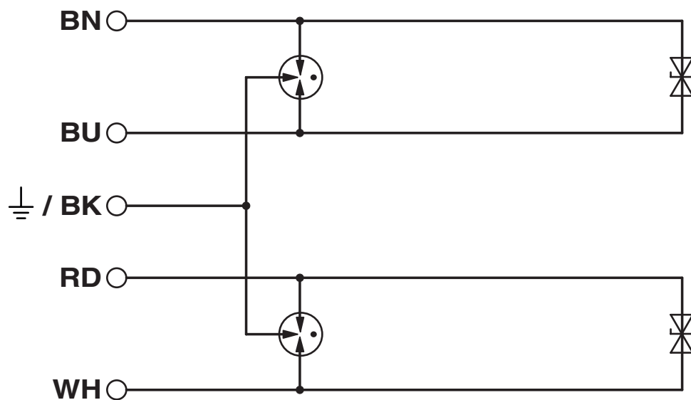
Diagrama eléctrico
