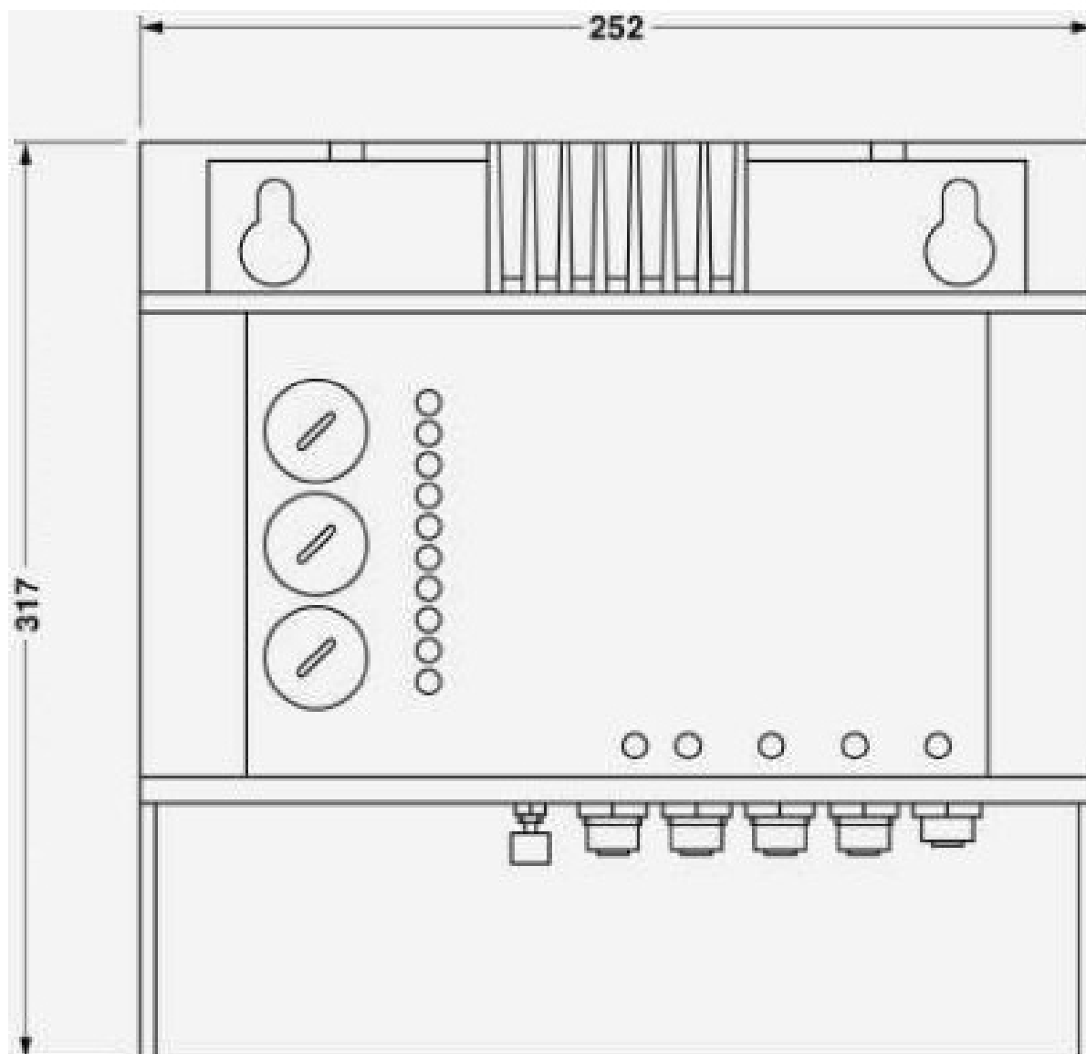
Esquema de dimensiones
