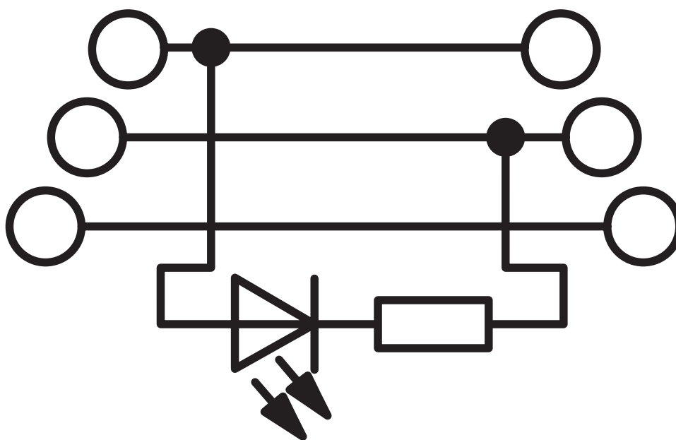
Diagrama eléctrico
