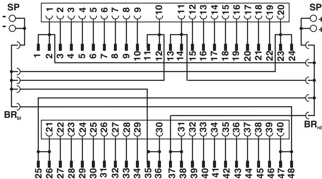
Diagrama eléctrico
