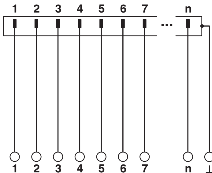
Diagrama eléctrico
