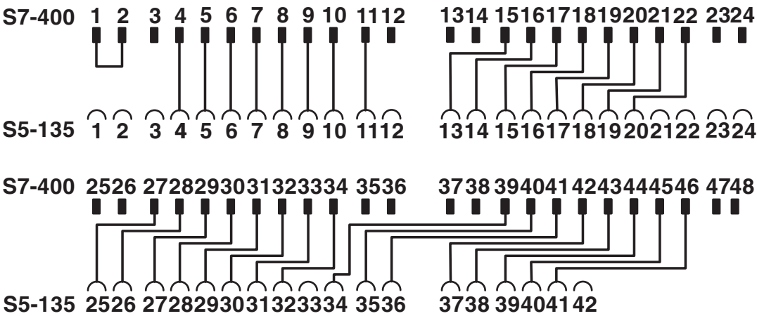
Esquema de conexiones FLKM S135-431-UA/S400
