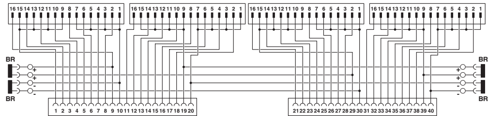
Diagrama eléctrico
